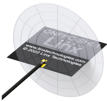
XZ-Plane Gain
